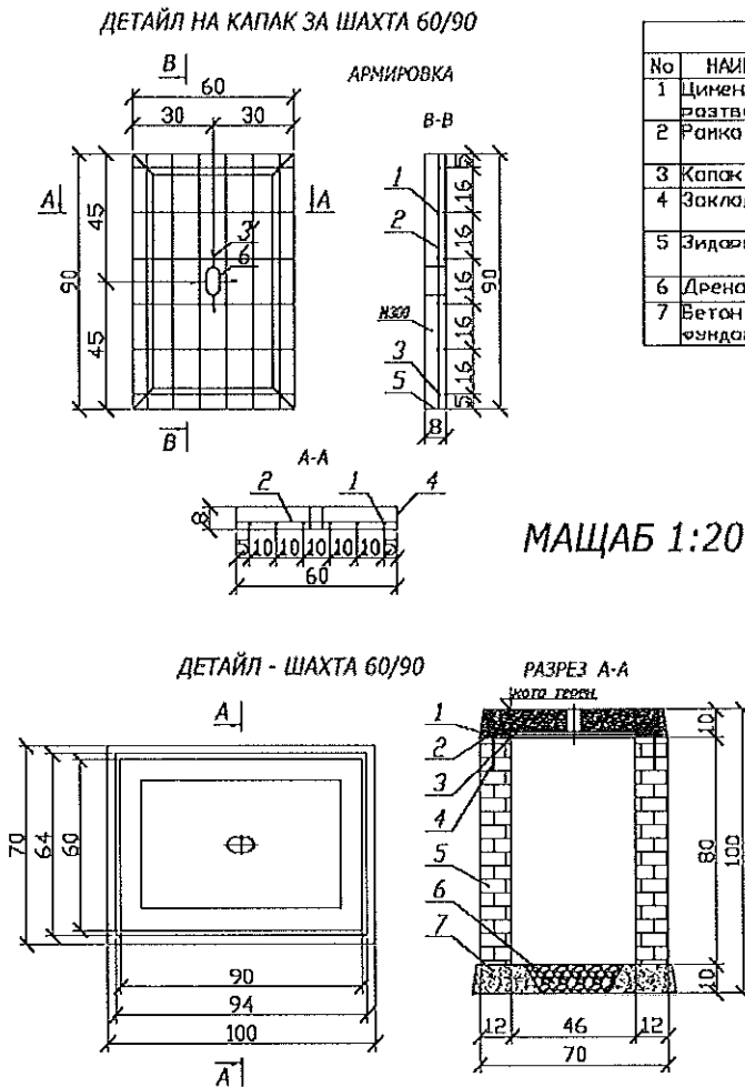
Фиг. 7.3. Кабелна шахта – единична
